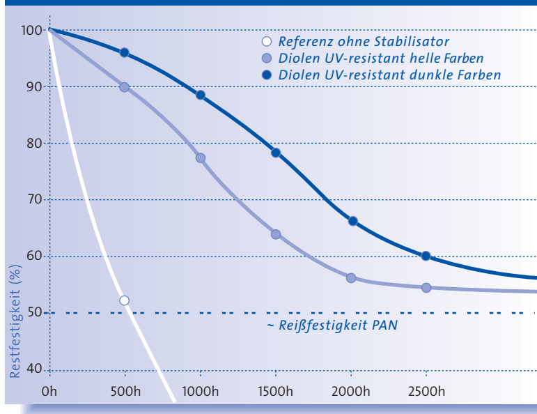
Diolen® UV-resistent im Vergleich zu Standard-PES Mechanische Prüfung (bewittert nach DIN EN 105 B04)
